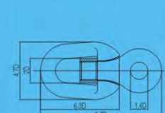
SWIVEL=SW(转环)
