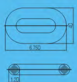
STUDLESS LINK=SL (无档环)
